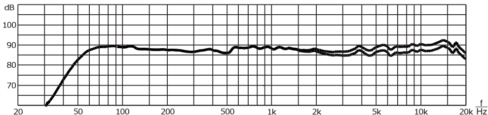
② Respuesta de frecuencia
